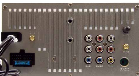
Anschlüsse des ESX VMX700DAB
